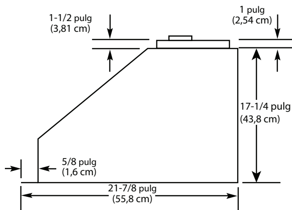
Instalación de ventilador 900, 1200 o 1500 CFM exterior o en línea
