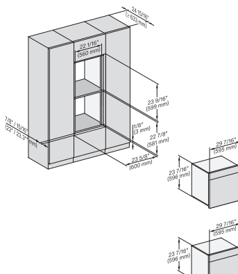
DGC786x, H7x6xBP, Einbau, 30 Zoll, Flush inset, combi, XXL 650S
