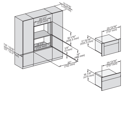
DGC7x4+EBA7848, H7x70BM(X), Einbau, 30 Zoll, Flush inset, combi, XL
