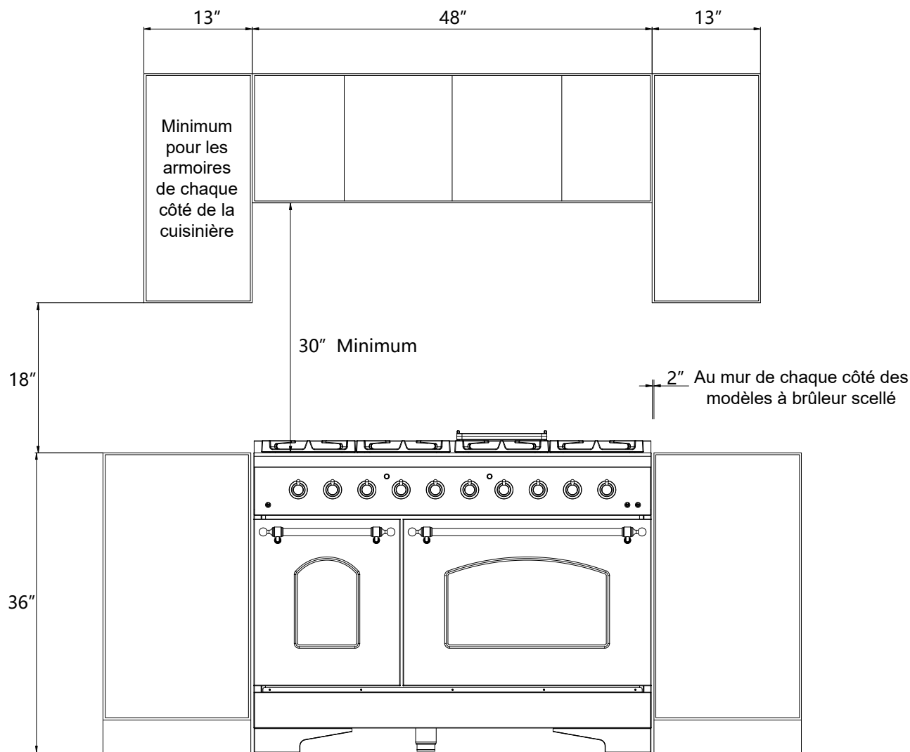
Diagramme d'installation
