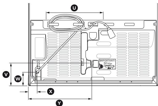
Dimensions des connexions en eau et 110VAC
