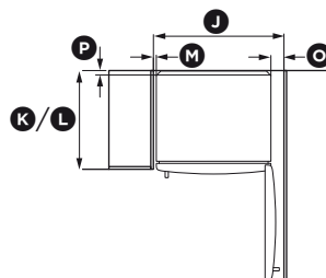
Porte du réfrigérateur au même niveau que l'armoire – ouverture de la porte à 90°
