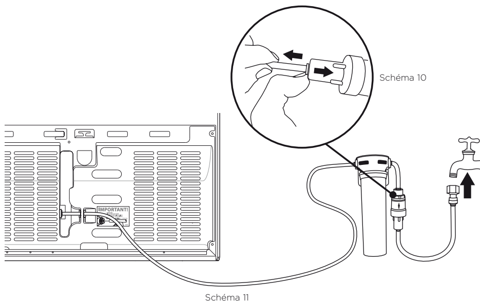
Raccordement au système d'alimentation en eau
